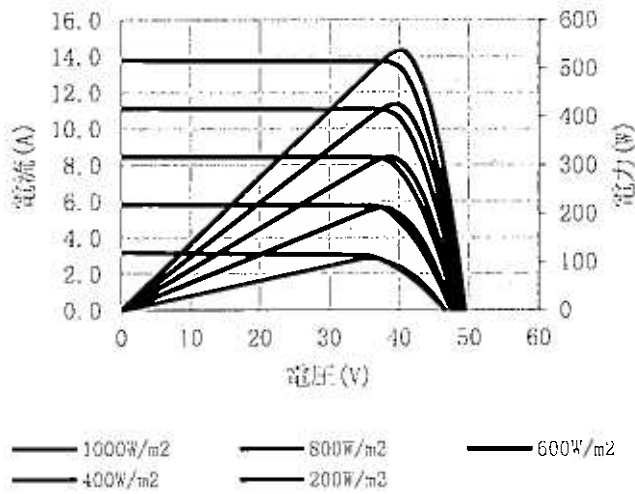
電流-電圧 & 電力-電圧曲線
