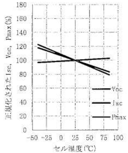
Isc, Voc, Pmax温度依存性
