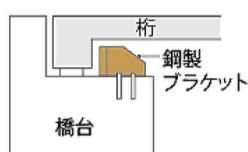
鋼製ブラケット突起構造工法
