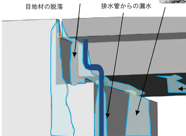
橋台の漏水
